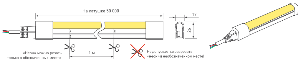
Рисунок 1. Габариты ленты «гибкий неон».
