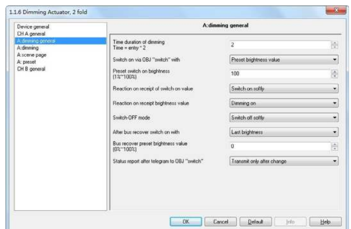
Fig. 6.4 Parameter window "CH X dimming general"
