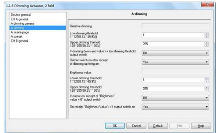
Fig. 6.5 Parameter window “X: dimming”
