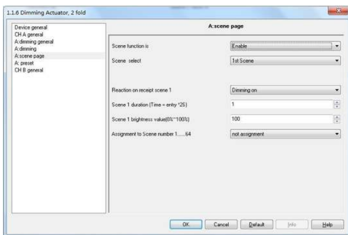
Fig. 6.6 parameter window "X: scene page"
