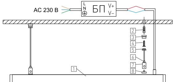
Рис. 2. Монтаж светильника
