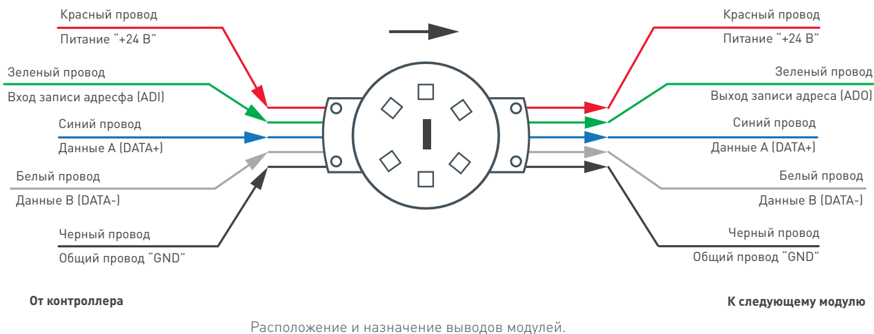
Расположение и назначение выводов модулей.
