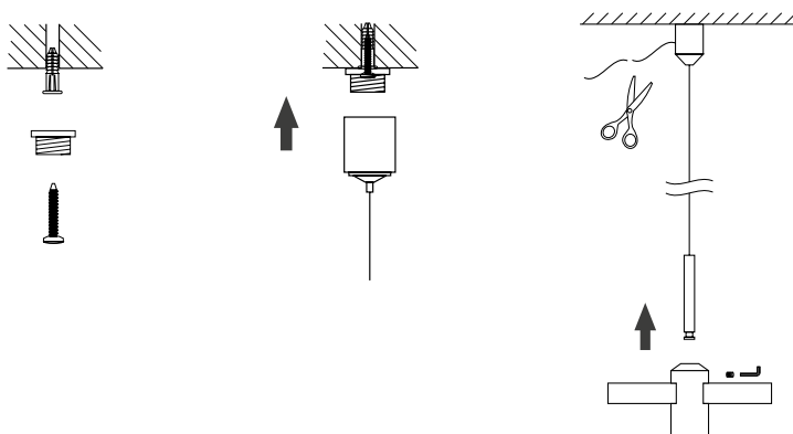
Рис. 2. Установка подвеса
