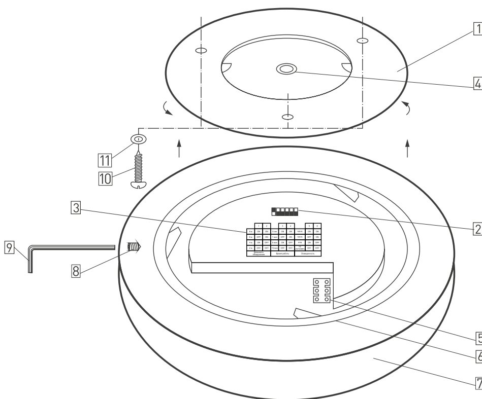
Рис. 3. Конструкция светильника
