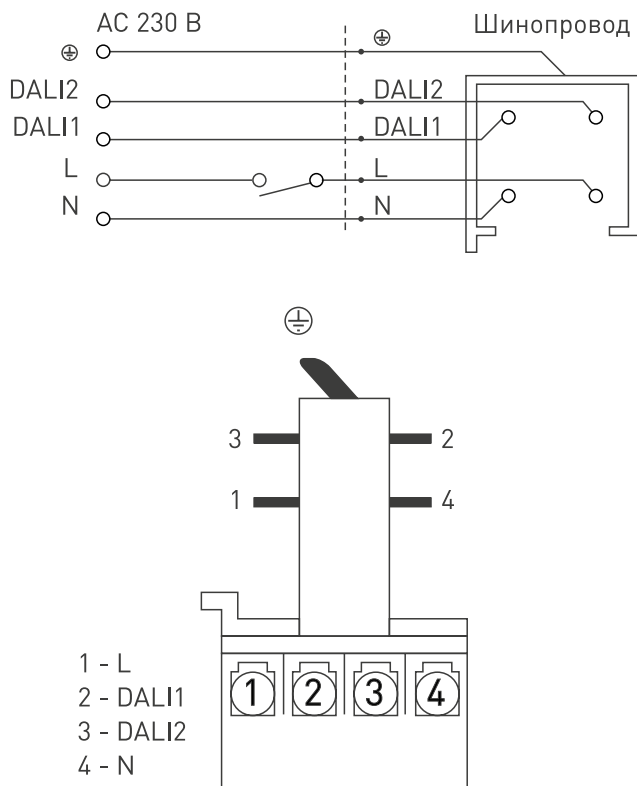
Рис. 2. Схема подключения
