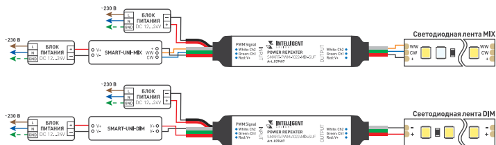
Рис. 1. Схема подключения усилителя SMART-PWM-1022-MIX-SUF
