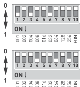
Рис. 2. DIP-переключатели
