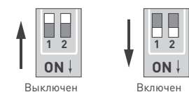
Рис. 3. DIP-переключатели терминатора
