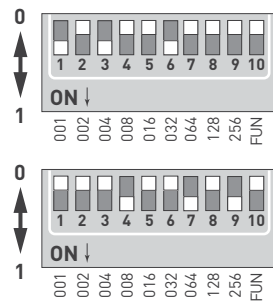
Рис. 2. DIP-переключатели
