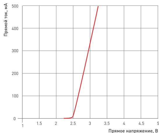
Зависимость прямого тока от прямого напряжения
