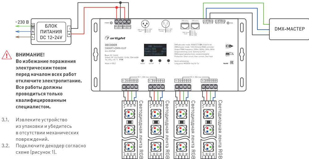
Рисунок 1. Схема подключения декодера SMART-DMX-SUF
