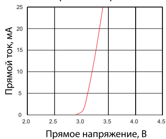
Зависимость прямого тока от прямого напряжения
