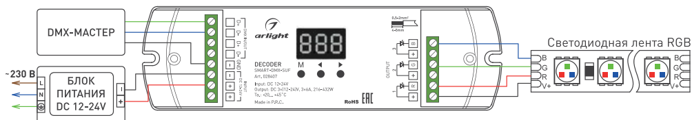
Рисунок 1. Схема подключения декодера SMART-DMX-SUF
