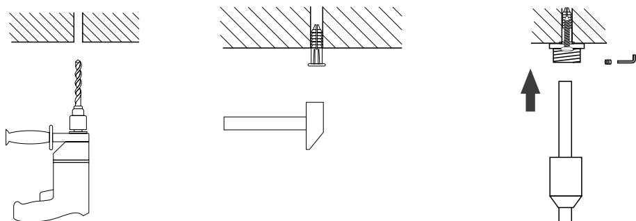
Рис. 2. Установка подвеса на поверхность и шинопровод
