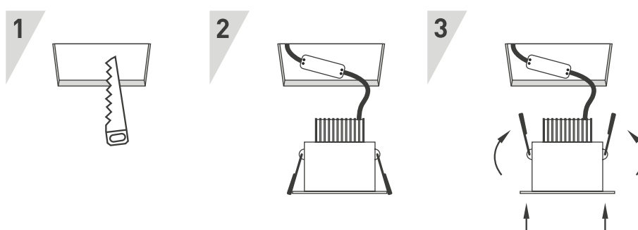
Рис. 2. Установка и подключение светильника
