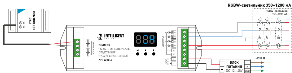
Рис.1. Пример схемы подключения диммера к светильникам (светодиодным модулям)
