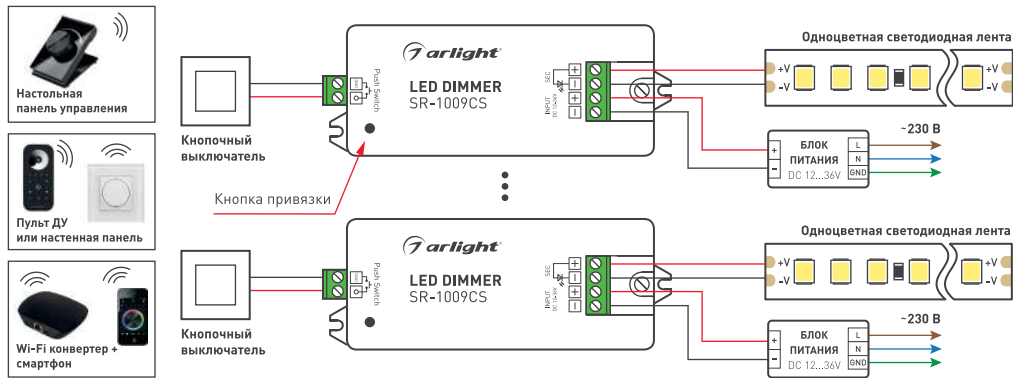
Рисунок 2. Схема подключения оборудования на примере диммеров SR-1009CS.
