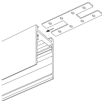
Рис. 4. Установка соединителей в пазы шинопровода
