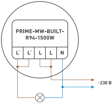
Рис. 2. Схема подключения датчика
