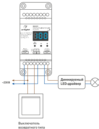
Рисунок 1. Схема подключения диммера SMART-D19-DIM-PUSH-DIN
