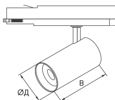
Рисунок 1. Чертеж и габаритные размеры
