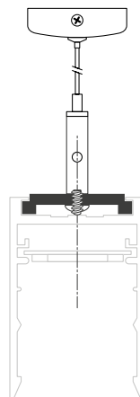
Рис. 1. Установка заглушек для системы MAG-25
