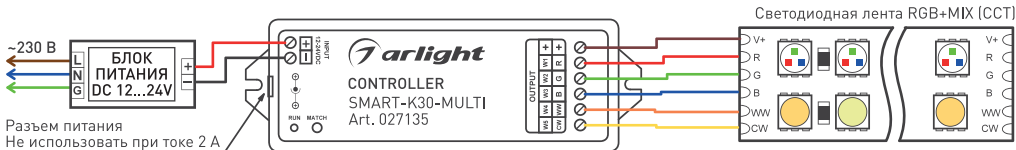
Рисунок 1. Схема подключения контроллера
