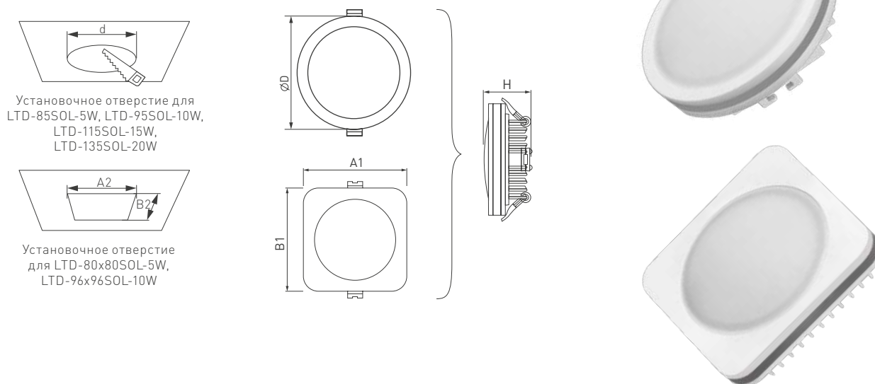
Рис. 1. Чертеж, габаритные и установочные размеры
