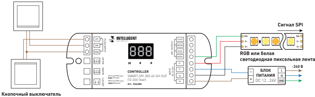
Рис. 2. Схема подключения выключателей возвратного типа (кнопки) к контроллеру
