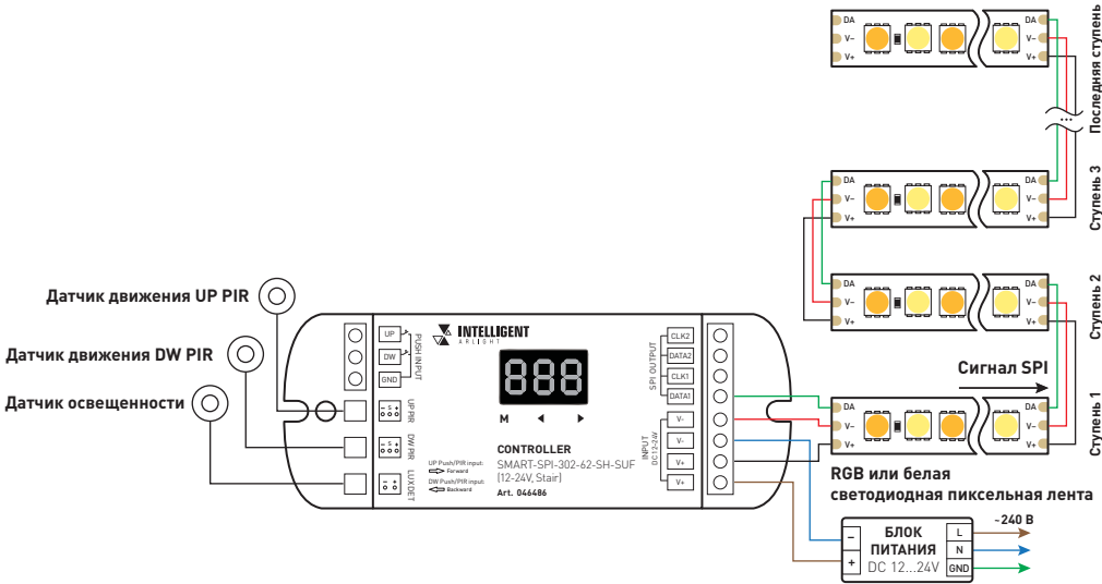
Рис. 3. Схема подключения контроллера для освещения ступеней лестницы
