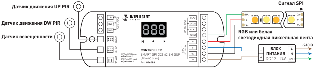
Рис. 1. Схемы подключения контроллера
