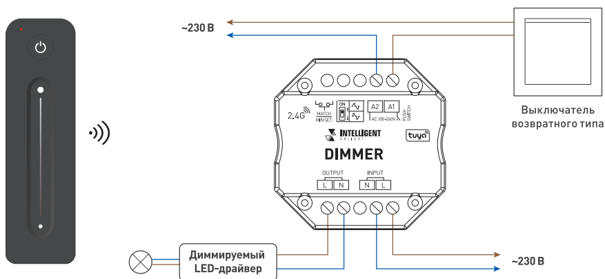
Рис. 1. Схема соединения оборудования
