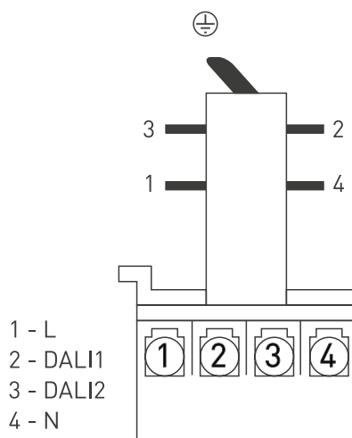
Рис. 2. Схема подключения
