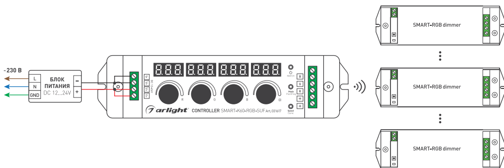
Рисунок 2. Схема подключения контроллера SMART-K60-RGB-SUF в режиме пульта дистанционного управления
