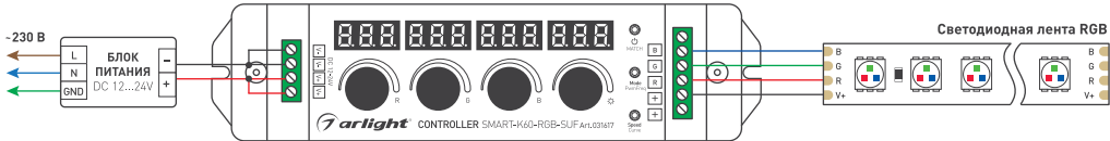
Рисунок 1. Схема подключения контроллера SMART-K60-RGB-SUF
