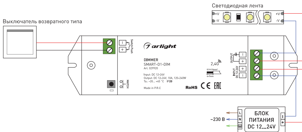
Рисунок 1. Схема подключения диммера SMART-D1-DIM
