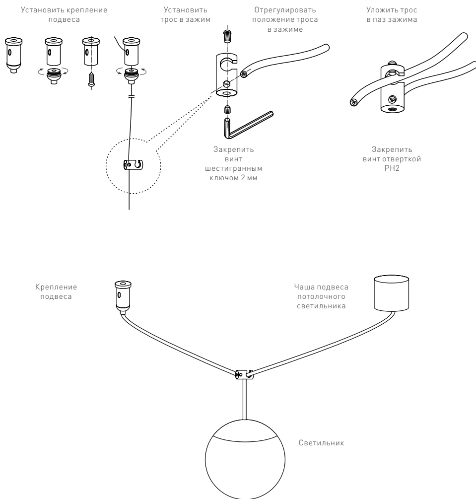
Рис. 1. Установка подвеса
