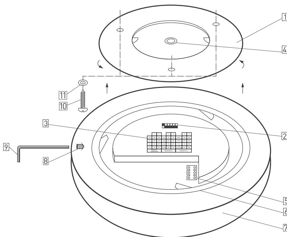
Рис. 3. Конструкция светильника
