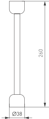
Рис. 1. Чертеж и габаритные размеры
