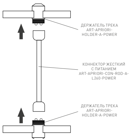
Рис. 2. Установка коннектора
