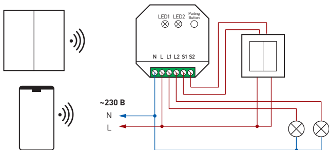
Рис. 1. Пример схемы подключения релейного модуля TY-702-72-WTI-WTO-PS-IN
