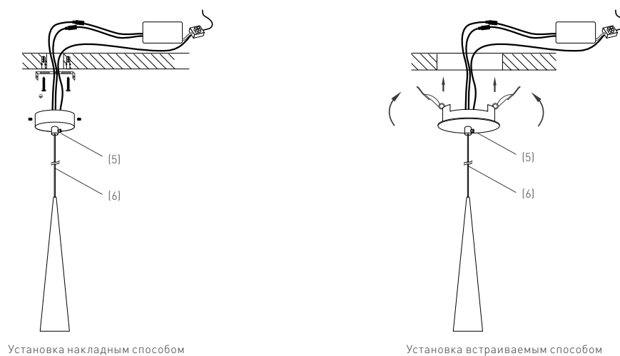
Рис. 3. Установка и подключение светильника
