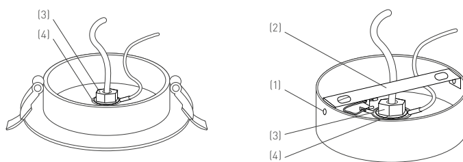
Рис. 2. Замена встраиваемой чаши на накладную
