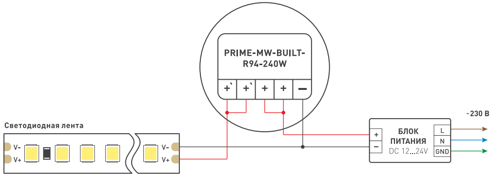
Рис. 2. Схема подключения датчика
