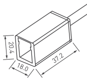
ARL-MOONLIGHT-1712- CON-POWER-HR-WH Арт. 028051
