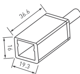
ARL-MOONLIGHT-1213- CON-POWER-HR-WH Арт. 028057
