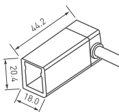
ARL-MOONLIGHT-1712- CON-POWER-LR-WH Арт. 028053
