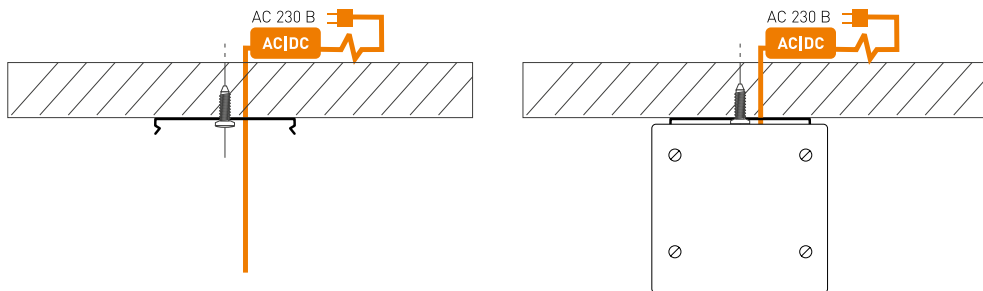
Рис. 1. Установка и подключение светильника
