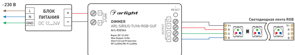
Рисунок 3. Пример схемы подключения диммера ARL-SIRIUS-TUYA-RGB-SUF
