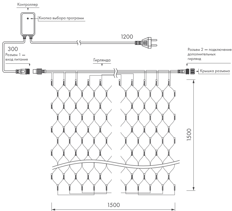
Рисунок 1. Схемы подключения
