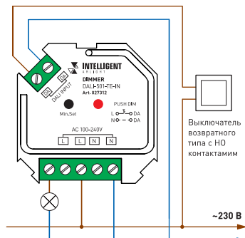
Рисунок 2. Схема подключения диммера
