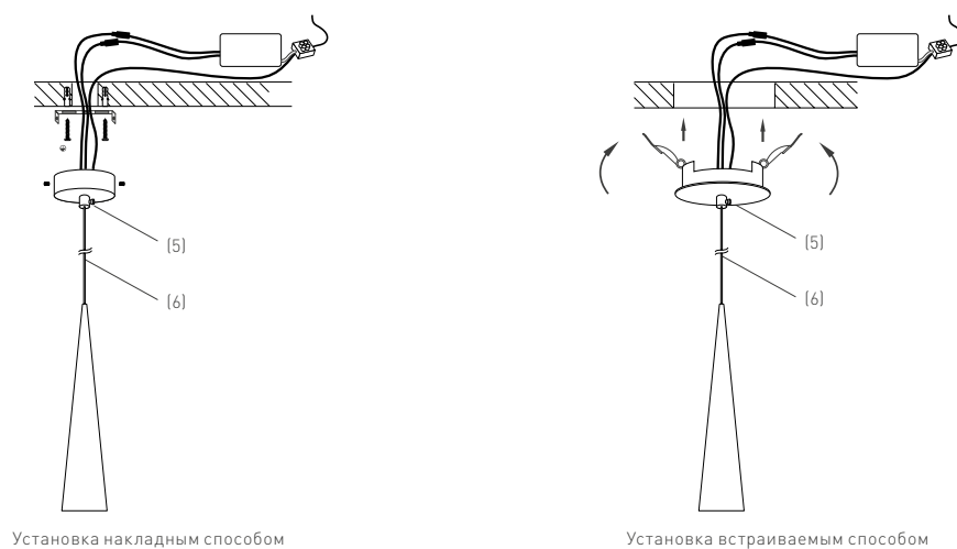
Установка накладным способом
