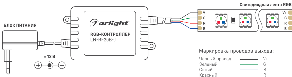
Рисунок 1. Схема подключения.
