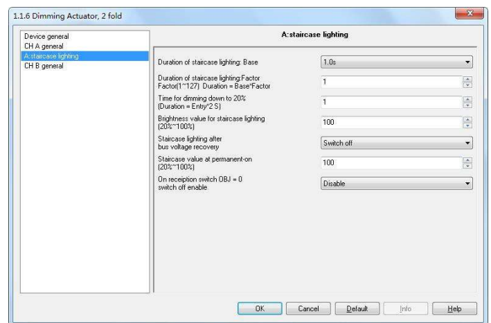
Fig. 2.7 parameter window “CH X staircase lighting”
