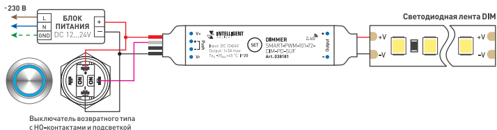
Рис. 2. Схема подключения диммера с использованием кнопки с подсветкой
