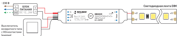
Рис. 1. Схема подключения диммера с использованием выключателя возвратного типа (кнопки)
