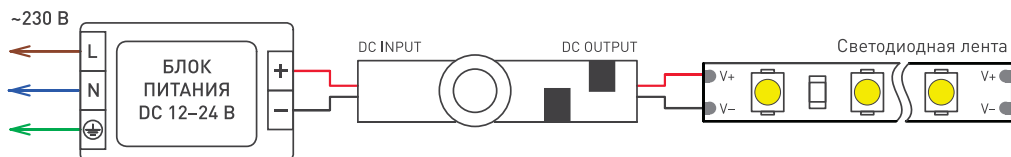
Рисунок 3. Схема подключения выключателя SMART-MOTION
