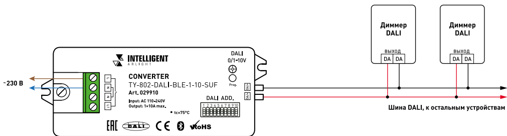
Рисунок 2. Схема подключения конвертера TY-802-DALI-BLE-1-10-SUF в режиме DALI.
