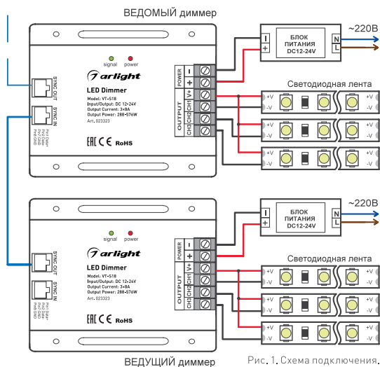
Рис. 1. Схема подключения.
