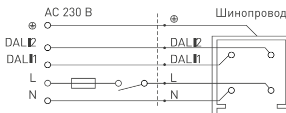
в) 1 фаза, 1 нагрузка, AC 230 В, 16 А, 1х3.7 кВА
