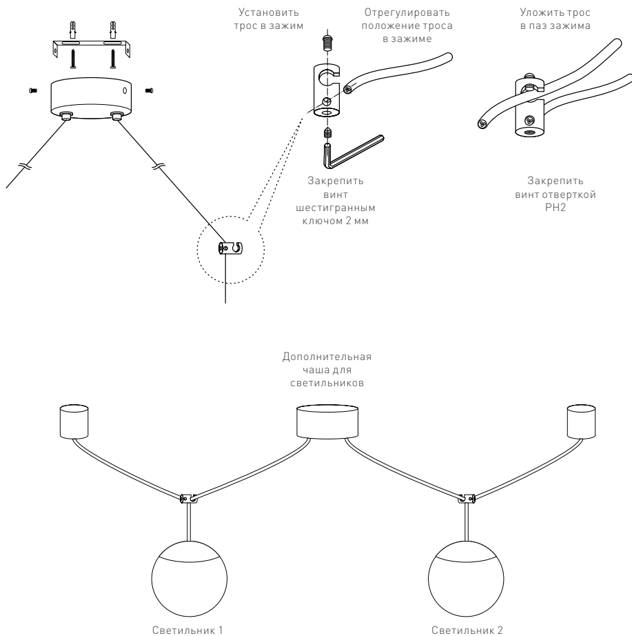
Рис. 1. Установка подвеса
